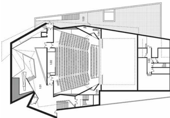
Grundriss 1. Obergeschoss • Floor plan first floor
